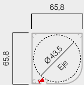
Perfil cajón 65 100153
